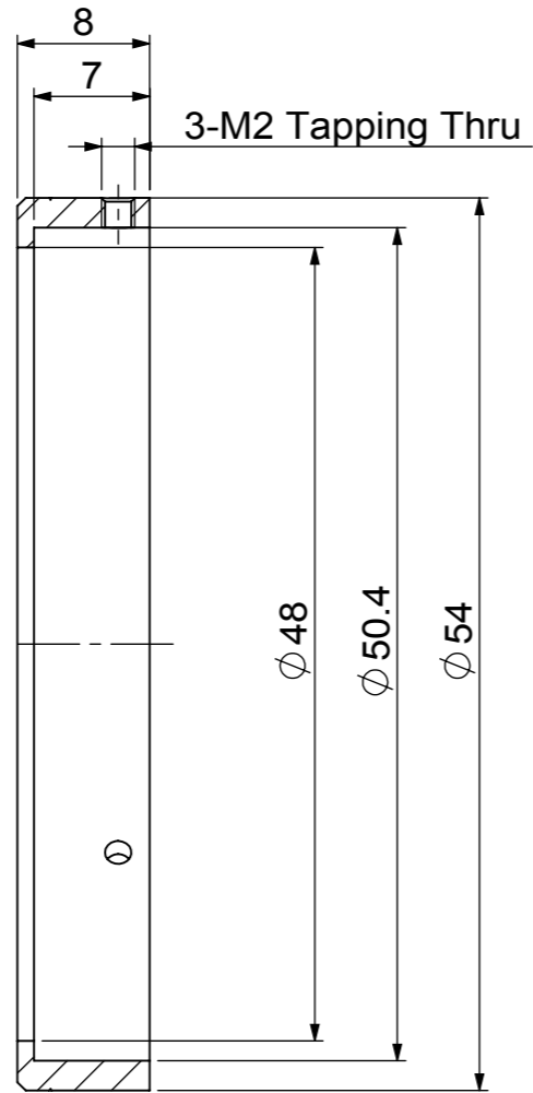
SECTION A-A
